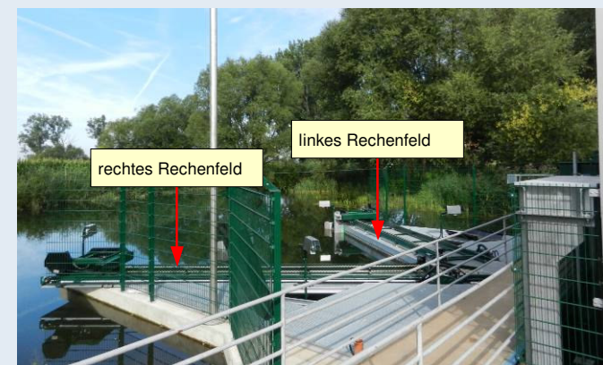
Seitenansicht des V-förmigen Horizontalrechens, Foto: L. Klauke
