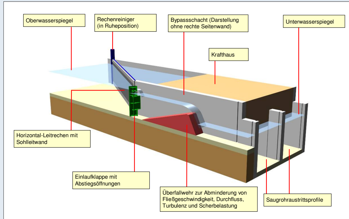
Prinzipskizze des Leitreechen-Bypass-Systems nach EBEL, GLUCH & KEHL (2001) in Seitenansicht
